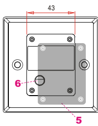
後視圖
