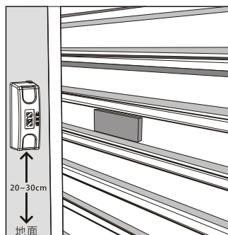
安裝的最佳距離 應離地20~30cm
