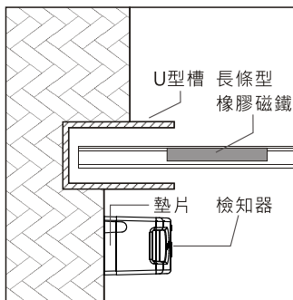
上視圖
