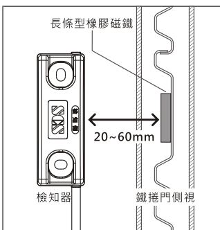
檢知器和橡膠磁鐵的 安裝間距應在20~60mm
