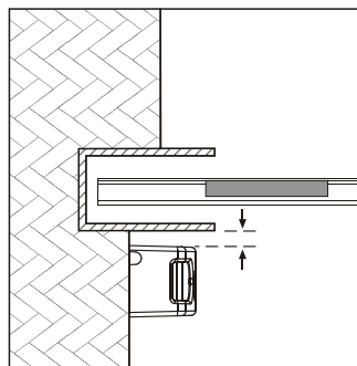
間距應大於10mm (太近會受到U型槽干擾)
