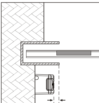
間距應小於5mm (高度不夠可加裝墊片)
