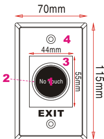
前視圖
