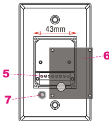
後視圖
