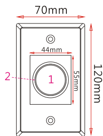
前視圖
