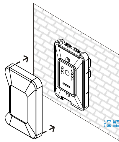
第三步：將外蓋閤上
