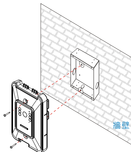
第二步：使用2顆螺絲將本體鎖在預埋盒上
