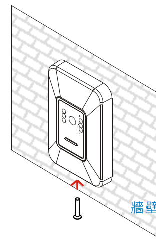
第四步：閤上後最後再鎖上下方的螺絲
